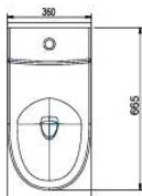
d4 Round Toilet Pan
